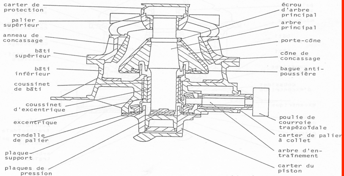
Concasseur Hydrocône Nomenclature des pièces
